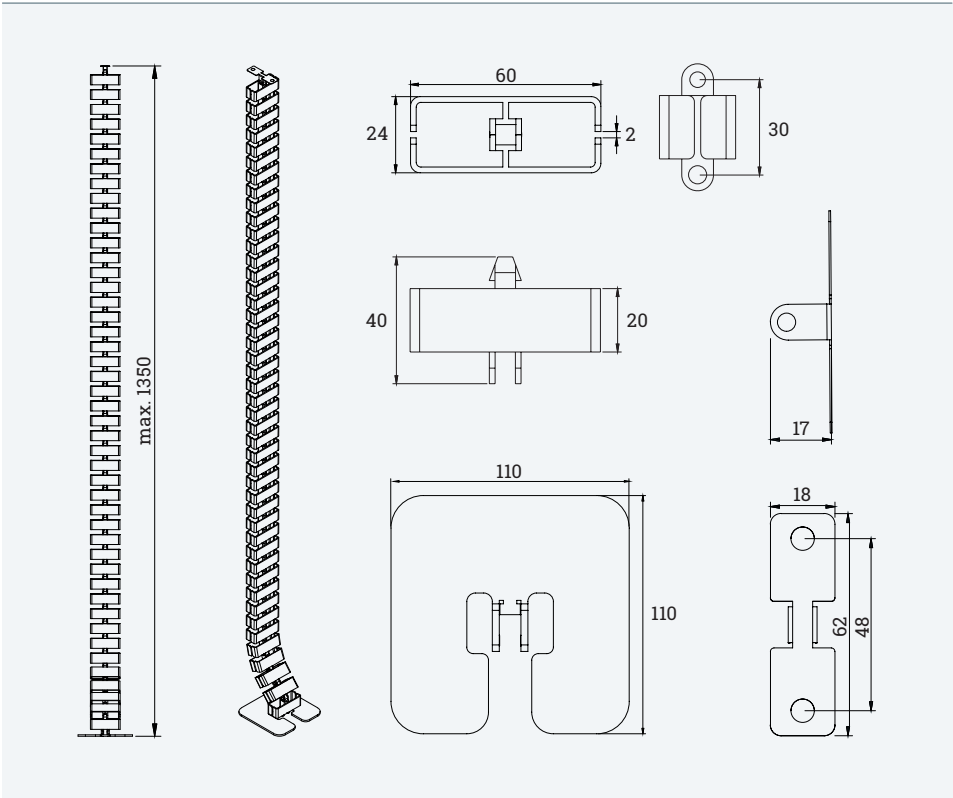
Fissaggio al piano tramite viti incluse
