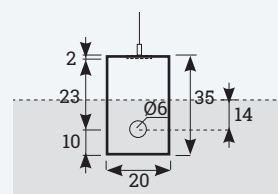
Schema di foratura sui pannelli AKUSTIX
