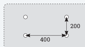
Schema di foratura sui pannelli AKUSTIX
