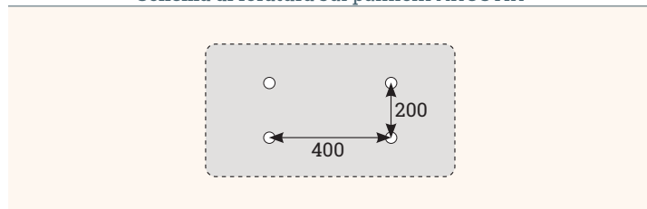
Schema di foratura sui pannelli AKUSTIX
