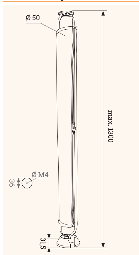
3 Base con peso per una maggiore stabilità
