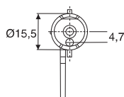
Ansicht von vorn Front view
