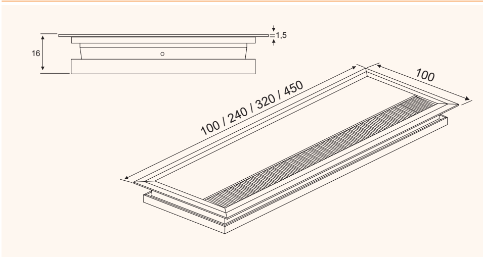
Disegni tecnici
