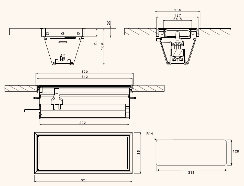
Disegni tecnici
