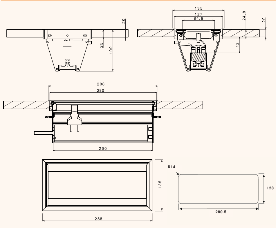
Disegni tecnici
